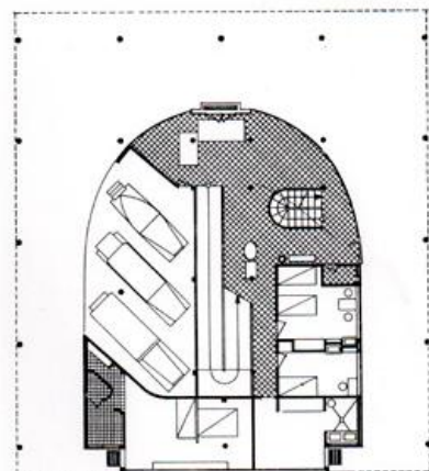
Villa Savoye. Plan du rez-de-chaussée. Poissy. 1929/1931
